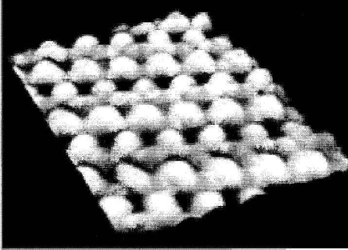
الجزيئية: بناء محكم من ذرات مترابطة ، عن موسوعة إنكارتا العلمية ٢٠٠٠
