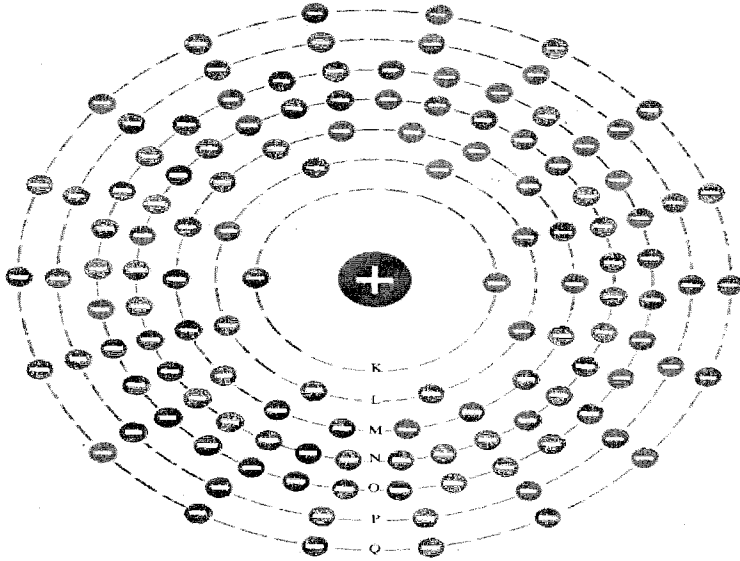
رسم توضيحي يبين تركيب الإلكترونات التي تحيط بالذرة
