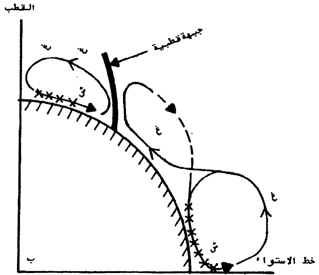
شكل ٢ (ب): الخلايا الثلاث اللاتي اقترحهن روسبي
