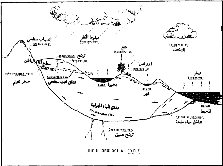
شكل ٢: الدورة المائية.
