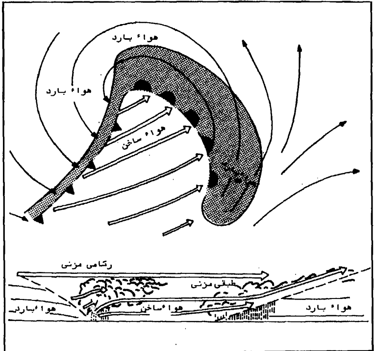
شكل ٧: الإعصار الموجي في مرحلة النضج
