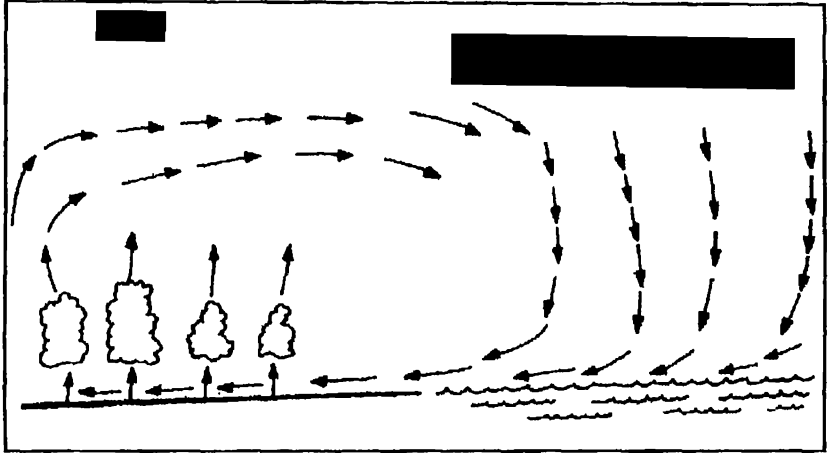
شكـل ١٠: رسم توضيحي للرياح... نسيم البحر ونسيم البر
