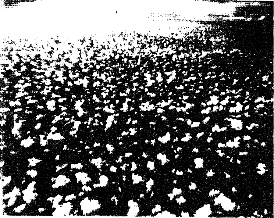
شكل ٤: تبين الصورة سحباً ركامية متفرقة تتجه ناحية منطقة تجمع في الأفق حيث يظهر سحب ركامي مزني.
