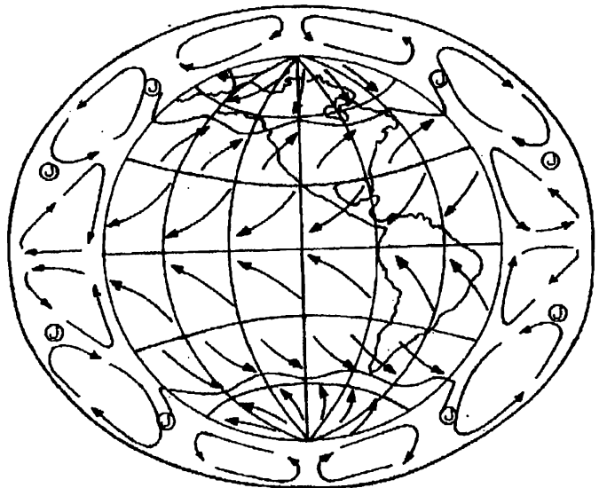
شكل ٣: رسم توضيحي للدورة العامة يظهر خلايا روسبي والرياح الشرقية والغربية.
