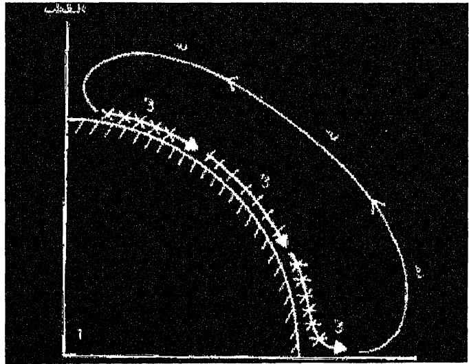
شكل ٢ (أ): الدورة العامة الشمالية الجنوبية وخلية هادلي (١) تبين الخلية الواحدة التي اقترحها جورج هادلي
