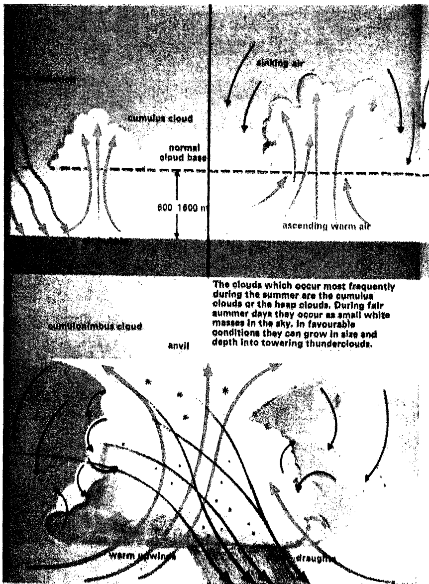
شكل ٧ - (أ، ب) : التيارات الصاعدة والهابطة داخل السحاب الركامي المنزني.
