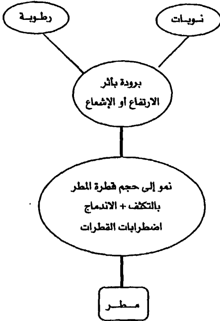
الشكل ٢ - خطوات عملية تكون المطر.
