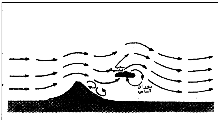
شكل ١١ (ب): حركة الرياح تظهر بوضوح الطابع الحلزوني حركة الهواء.
