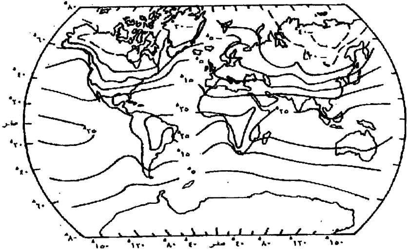
شكل ٥: متوسط التوزيع الحراري في يناير
