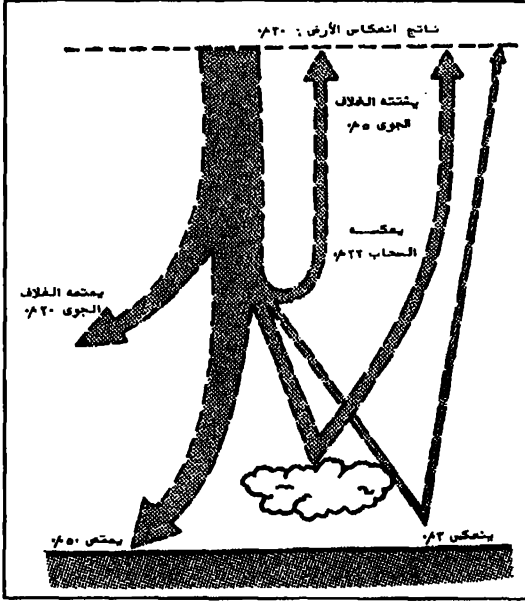
شكل ٤: التوازن الشعاعي للأرض
