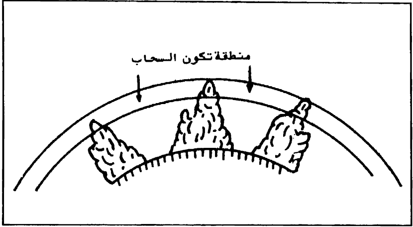
شكل ٢: نظرية أرسطو في تكوين السحاب على قمم الجبال.
