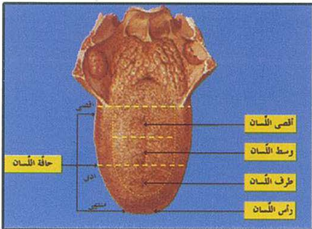
أقسام اللسان
