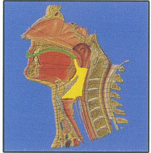
تجويف الفم
