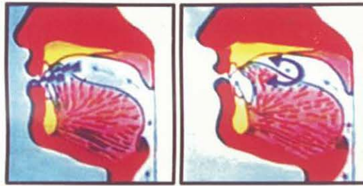
الراء
