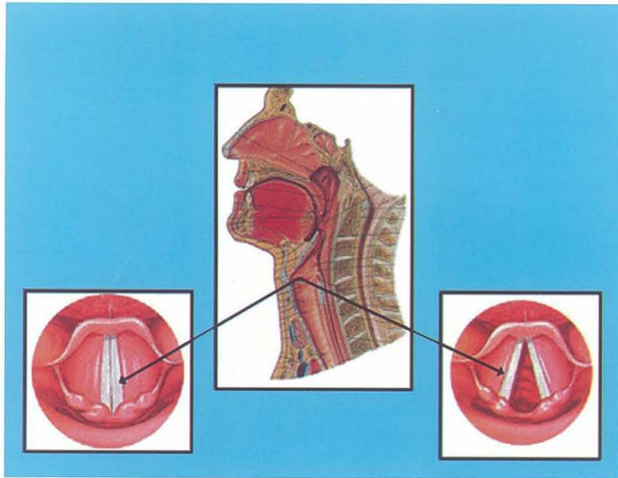
حالة الجهر
