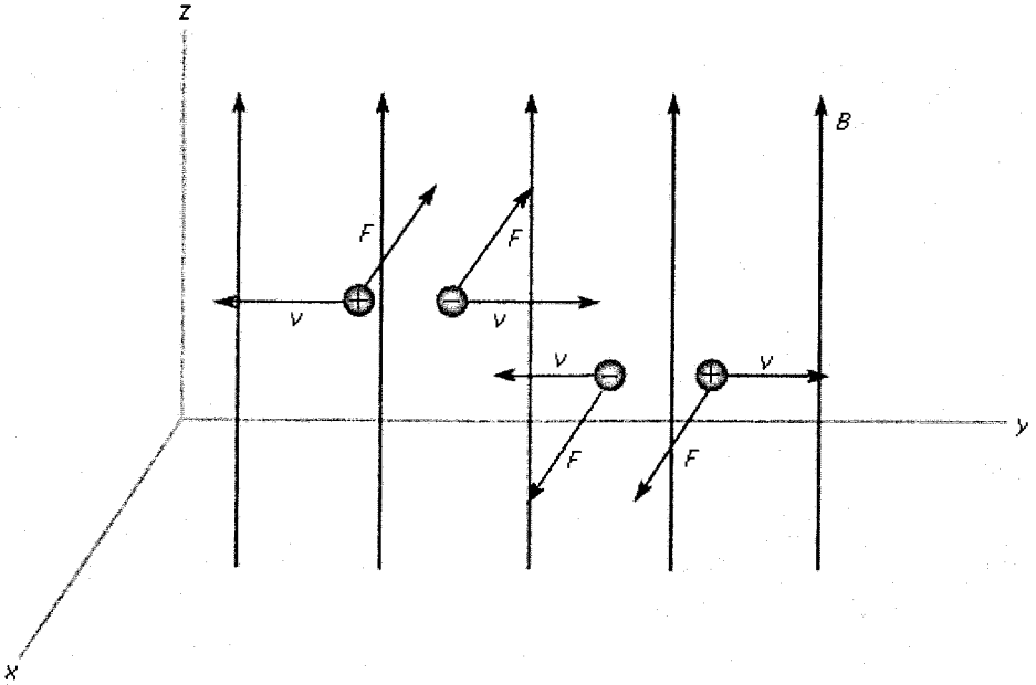
شكل يوضح القوة المغناطيسية لدقائق مشحونة متحركة
