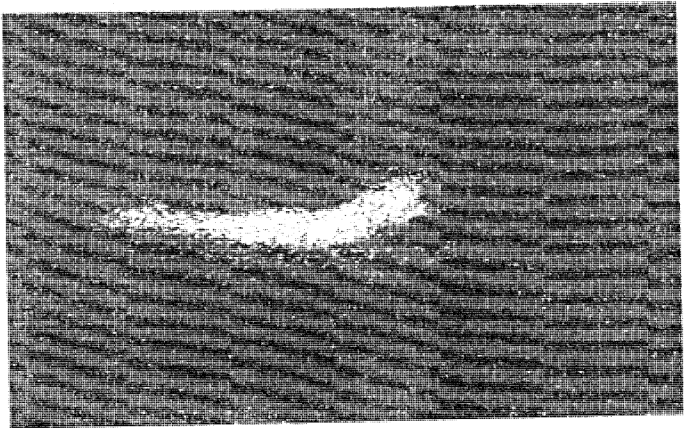
شكل يوضح بنية معبزة ضمن خليط لداني - حديدي لسطح متآكل ضمن مادة أنبوب مطاطي - معني متكون من مادة لدان (PA٦٦) مع ٨% من (HDPE) غني بالحديد والنيكل (١.٥ Ni steel shaft). الشكل لداني يوضح انتشار وتوزيع الحديد - النقاط البيضاء - ضمن المادة في الشكل العلوي. عن كتاب أطلس أضرار اللدائن (لوثر ليكل، هيرمن كلنجل، جوتفريد إيهريتمون، هيلموت تشاير)، (ص ٥٩). التكبير ٢٠٠٠ مرة
