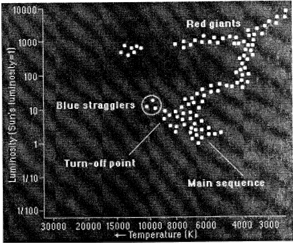
مخطط سيرنغ - رسل الذي يلخص حياة النجوم
