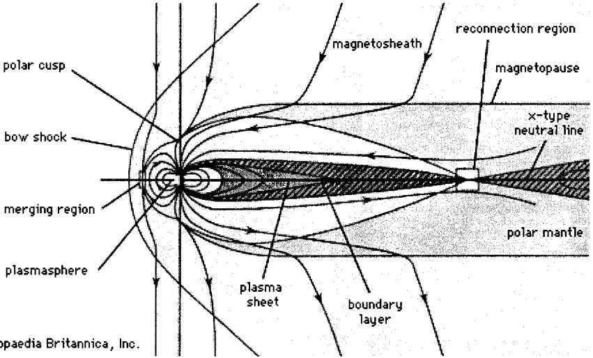
شكل يبين الطبقات التي يتشكل منها طبقة الماغنتوسفير ضمن الغلاف الجوي الأرضي
