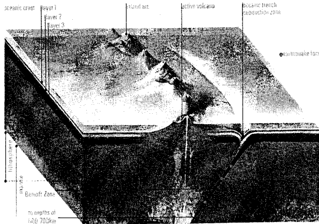
شكل: يوضح طبقات الأرض السطحية والتحتية، عن كتاب قاموس المصطلحات العلمية والفنية والهندسية، ص ١٩٣.
