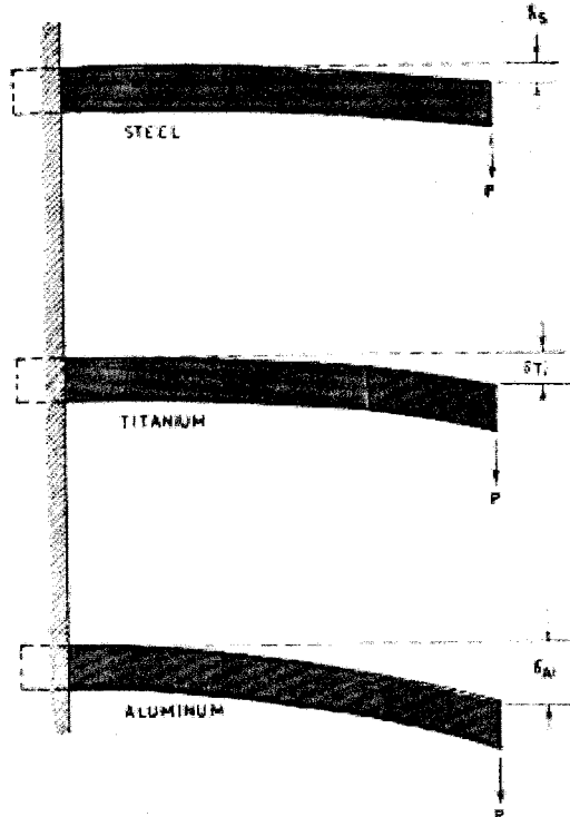
شكل يوضح قوة ومقاومة الحديد للشد والانحناءات أكثر من غيره من المعادن
