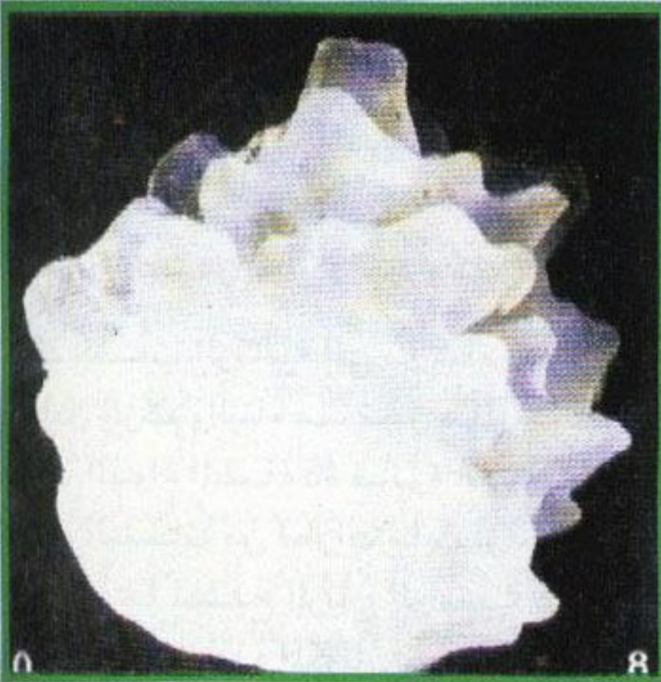
شكل (٥) : تبين الصورة قطعة برد سقطت خلال عاصفة ركامية مزنية ، يوضح المقياس أن قطرها حوالي ٨ سم
