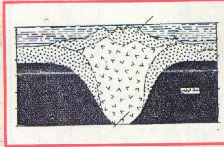
شكل (٢) يوضح جذراً بازلتيا من قشرة محيطية منفرد في طبقة الوشاح .
