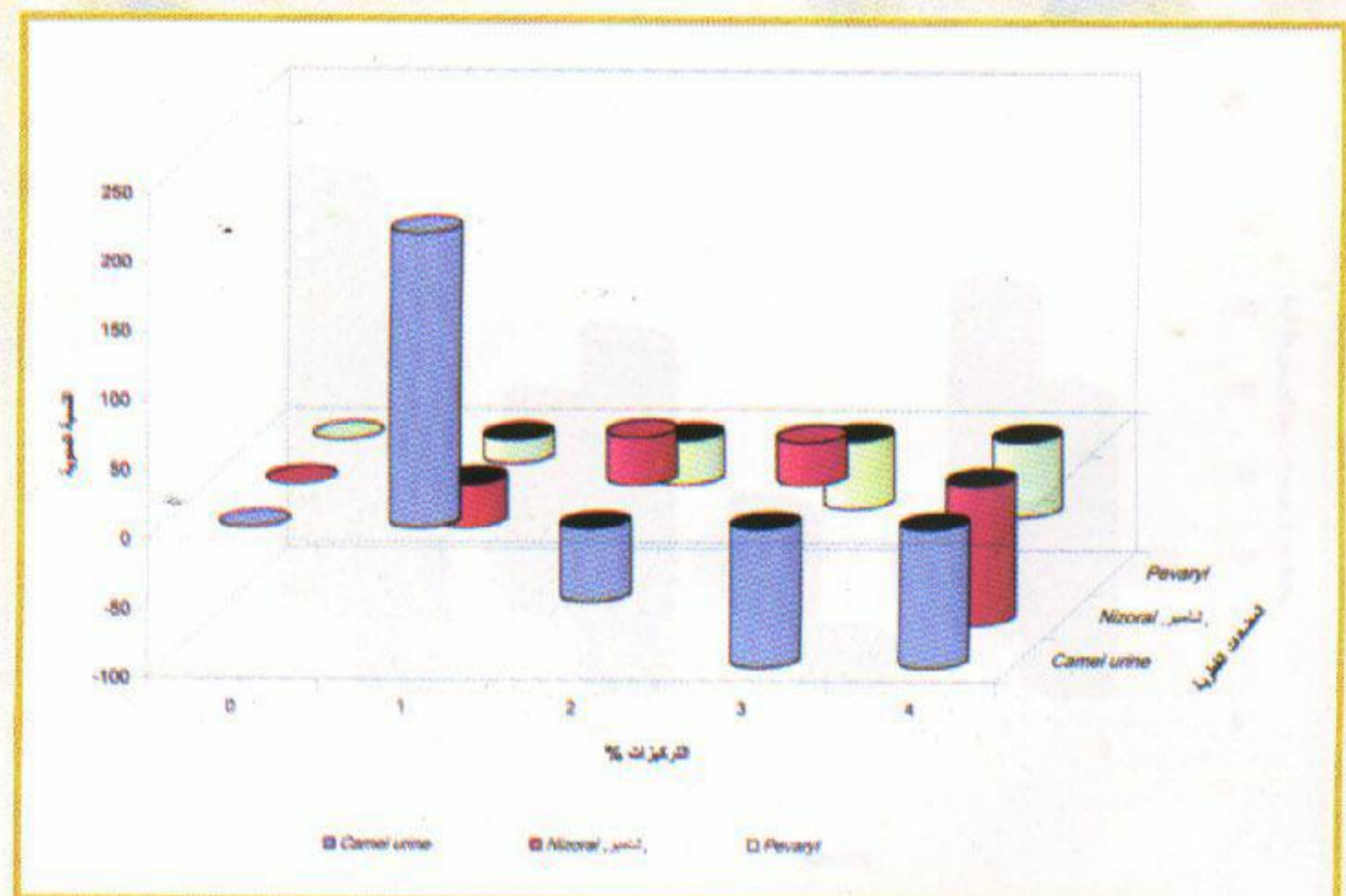
الوزن الجاف لفطر Aspergillus niger بعد المعاملة بتركيزات مختلفة من بول الإبل والمضادين للفطرين Pevary و Nizoral مقارنة بالعينة الضابطة
